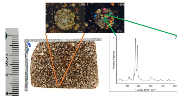
Analisi Raman di condruili in meteoriti
