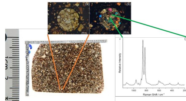
Analisi Raman di condriuli in meteoriti
